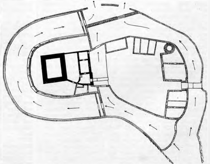
Schloss Hallwil im 14. Jahrh. Die Bauten des 12. Jahrh. sind tiefenschwarz gehalten. Nach Lithberg: Schloss Hallwil .
